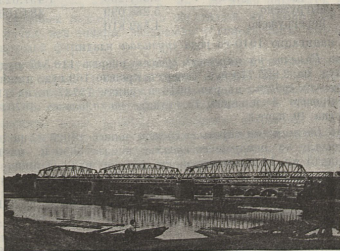
Ж.д. дор. мосты чрезъ р. Сожь.
